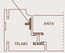
GUARNIZIONE TERMOESPANDENTE
